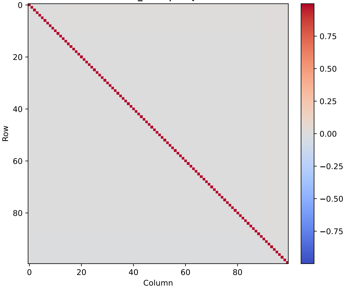
muon_zero | step 9
